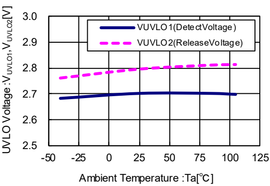
XC9267B75xxx
