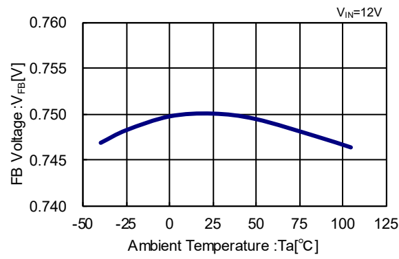
XC9267B75xxx
