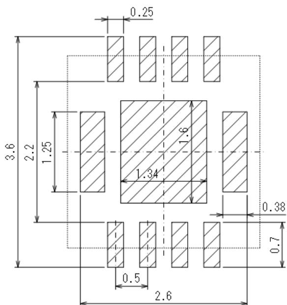
●参考パターンレイアウト/ Reference Pattern Layout
