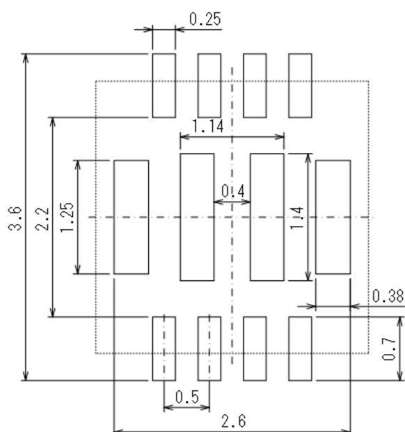
●参考メタルマスクデザイン/ Reference Metal Mask Design
