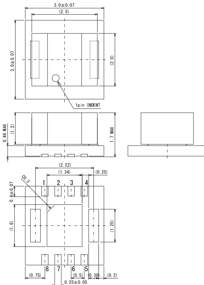
●参考メタルマスクデザイン/ Reference Metal Mask Design
