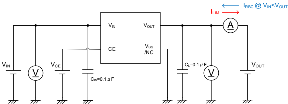
測定回路図③
