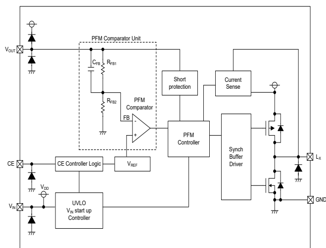
XC9265Axxx/XC9265Bxxx タイプ
