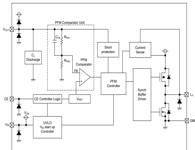
XC9265Cxxx/XC9265xxx タイプ
