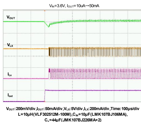
XC9265B301
